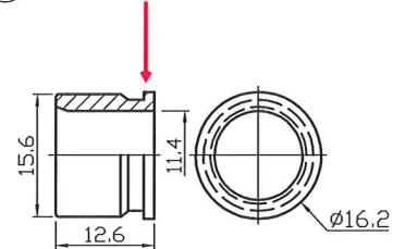
Ⓓ b) シール先端部の形状及び各部寸法 変更
