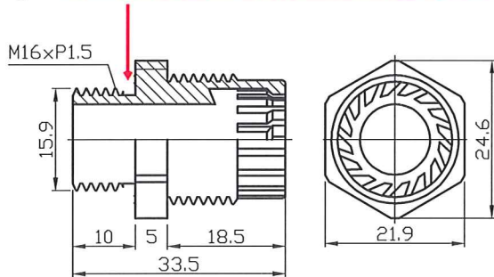
Ⓒ d) 本体取付ネジ部根元の形状及び各部寸法変更
